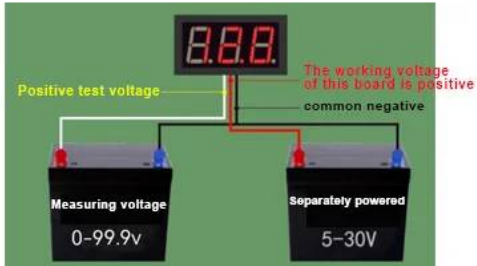
DC Digital Voltmeter
